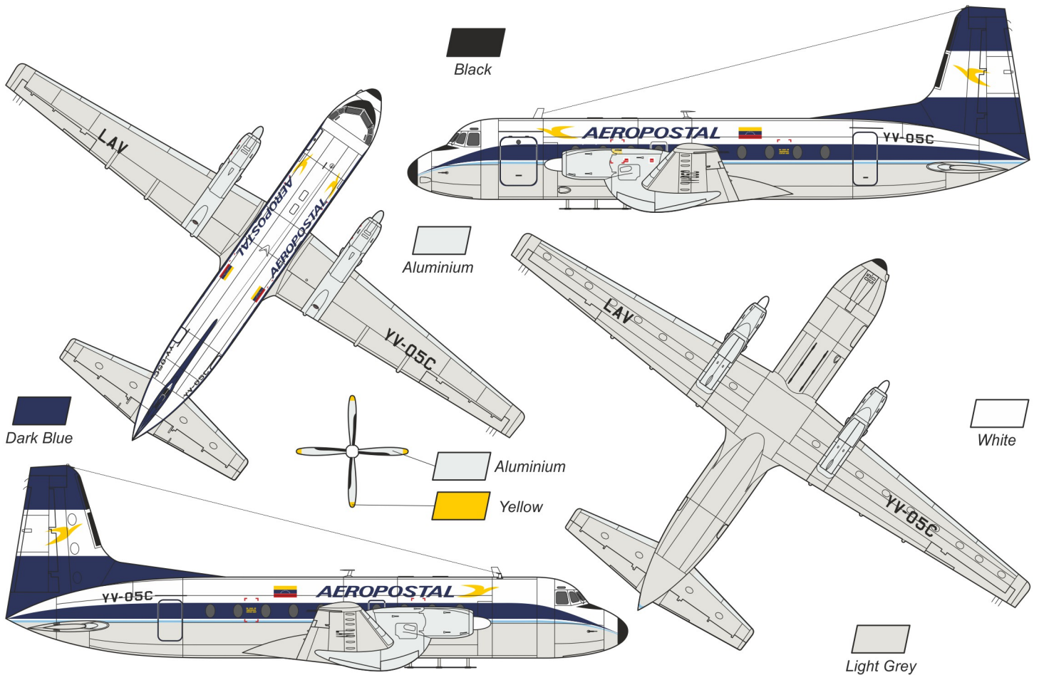
C Hawker Siddeley HS.748 (Srs.2 Model 215), YV-05C (c/n 1578), Línea Aeropostal Venezolana S.A. (LAV), Caracas - Simón Bolívar International Airport (Aeropuerto Internacional de Maiquetía "Simón Bolívar"), Venezuela, 1980-82
