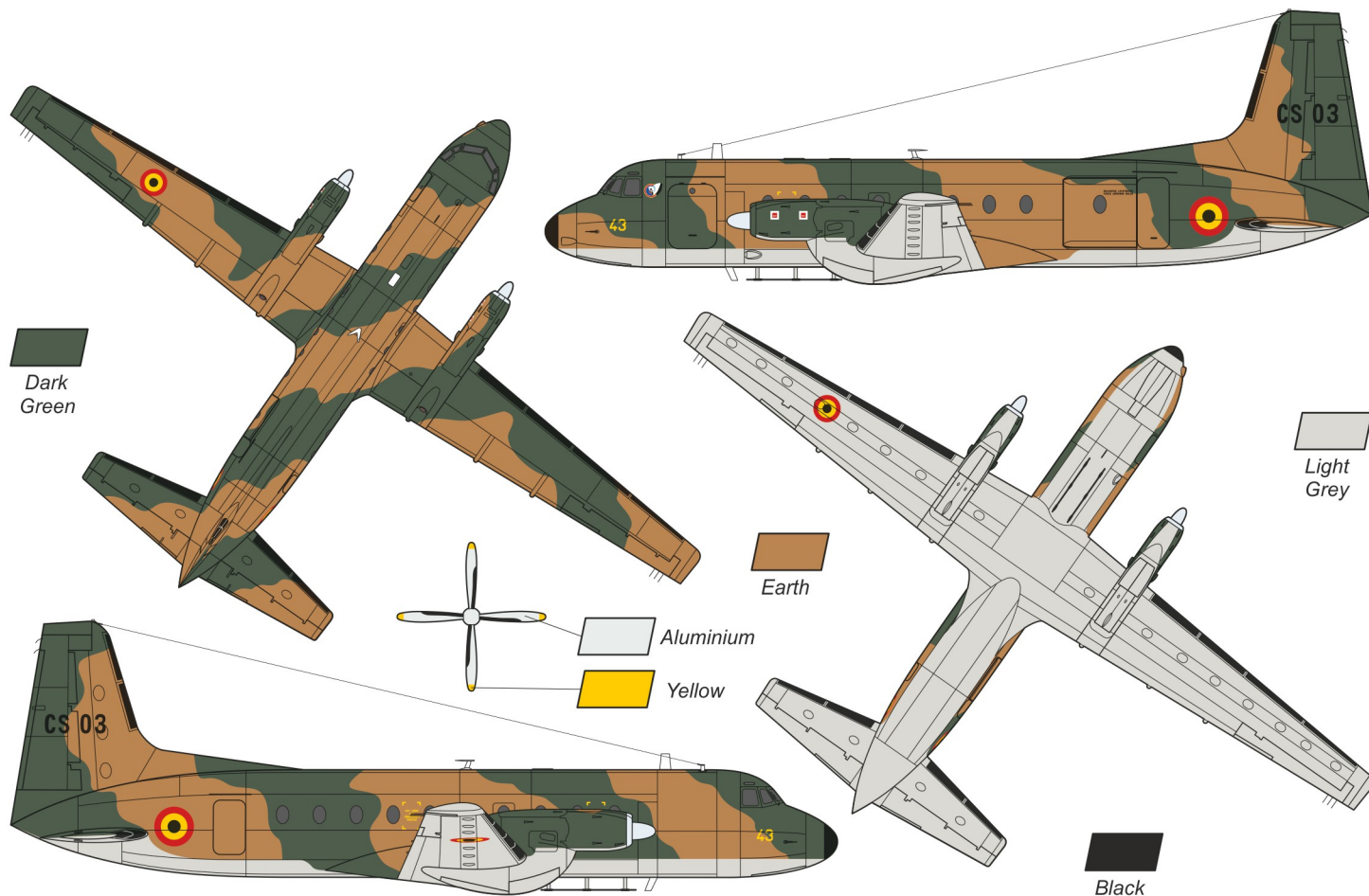
C Hawker Siddeley HS.748 (Srs.2A Model 288) Andover, CS-03 (c/n 1743), Yellow 43, 21° Esc. 'Sioux', 15° Wing Transport Aérien, Belgian Air Force (Force aérienne belge/Belgische Luchtmacht), Brussels/Melsbroek Air Base, Belgium, 1978
