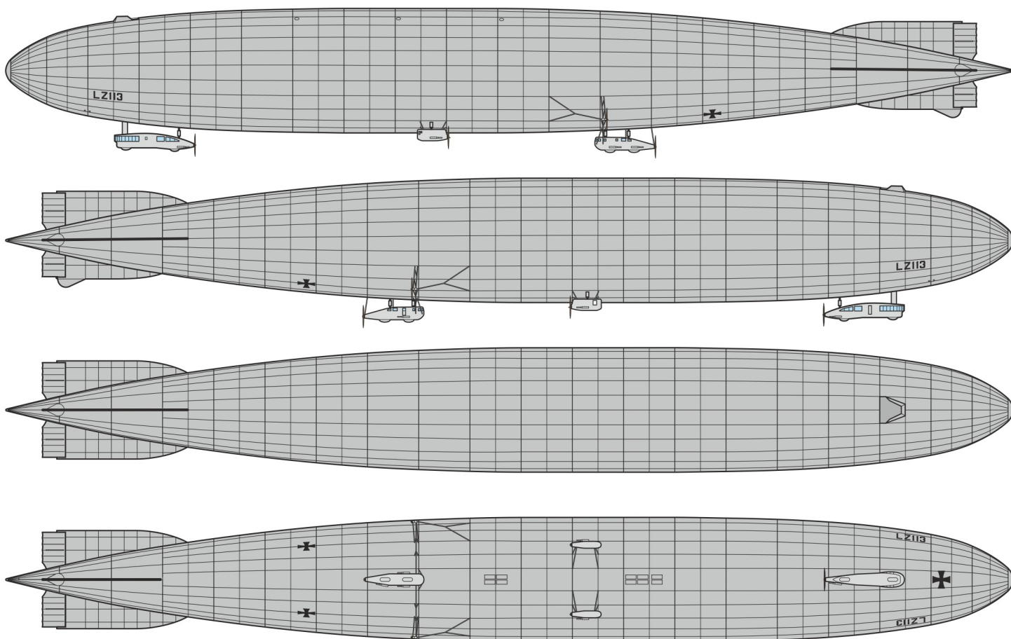
A Zeppelin LZ83 (R-class), LZ113, Black LZ113, Airship Troop (Luftschifftruppe), Imperial German Flying Corps (Fliegertruppe des deutschen Kaiserreiches), Seddin bei Stolp Airship Base, Germany, spring 1917
